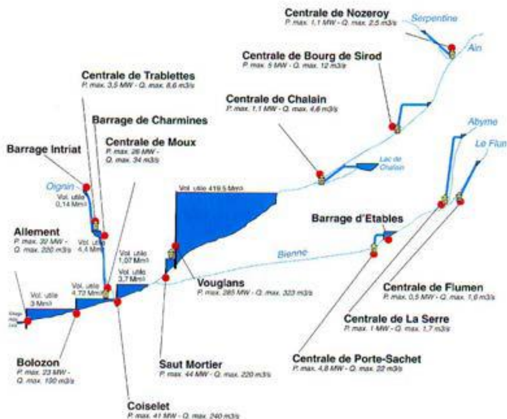
Figure K : Schéma récapitulant l'ensemble des barrages hydroélectriques et microcentrales exploités par EDF sur l'amont du bassin versant de la rivière d'Ain (Source EDF)
