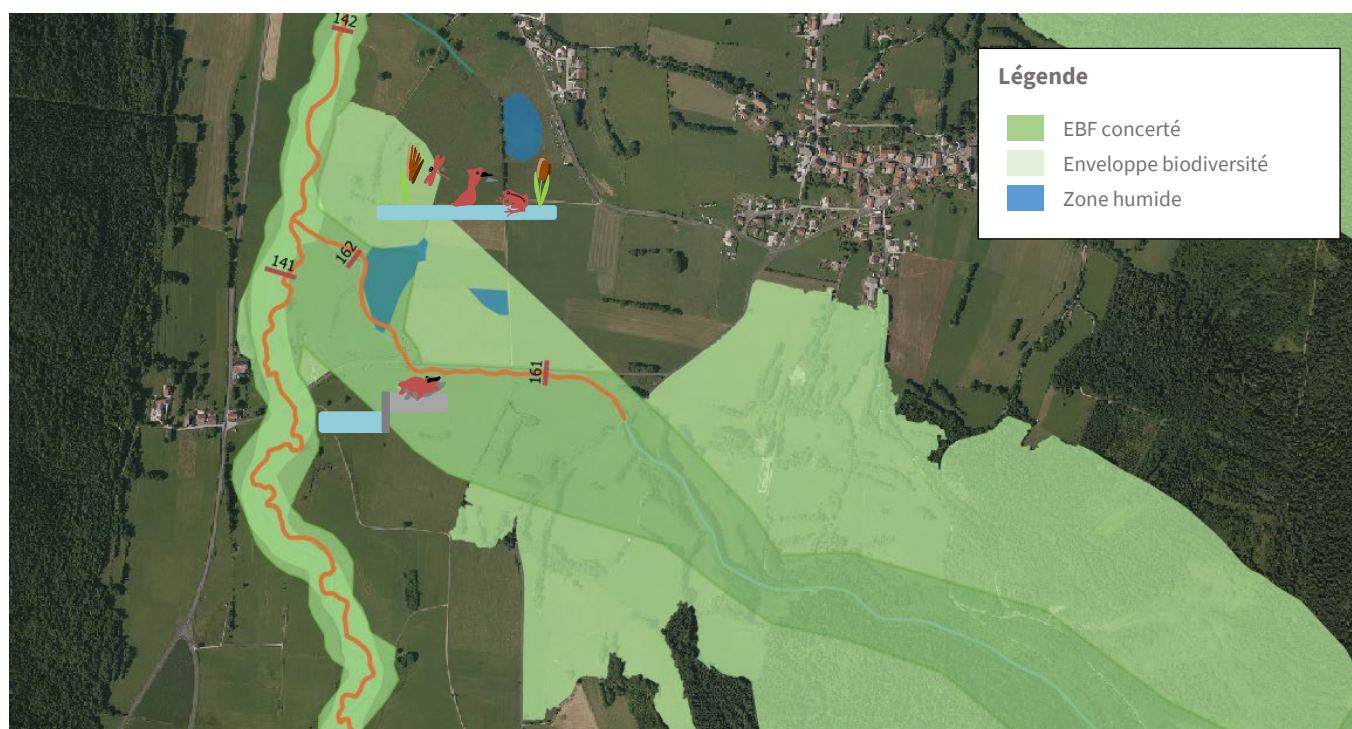
SCHEMA DE PRINCIPE D'UNE RESTAURATION D'UN COURS D'EAU R2
