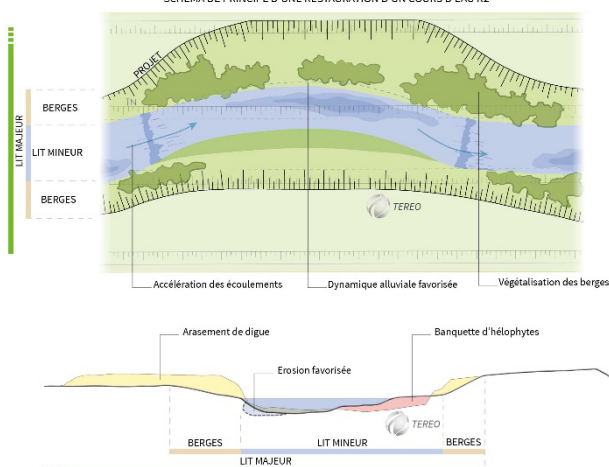
SCHEMA DE PRINCIPE D'UNE RESTAURATION D'UN COURS D'EAU R2
