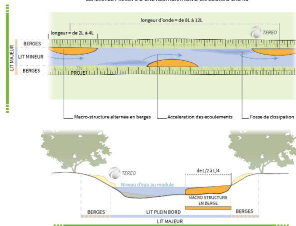
SCHEMA DE PRINCIPE D'UNE RESTAURATION D'UN COURS D'EAU R1
