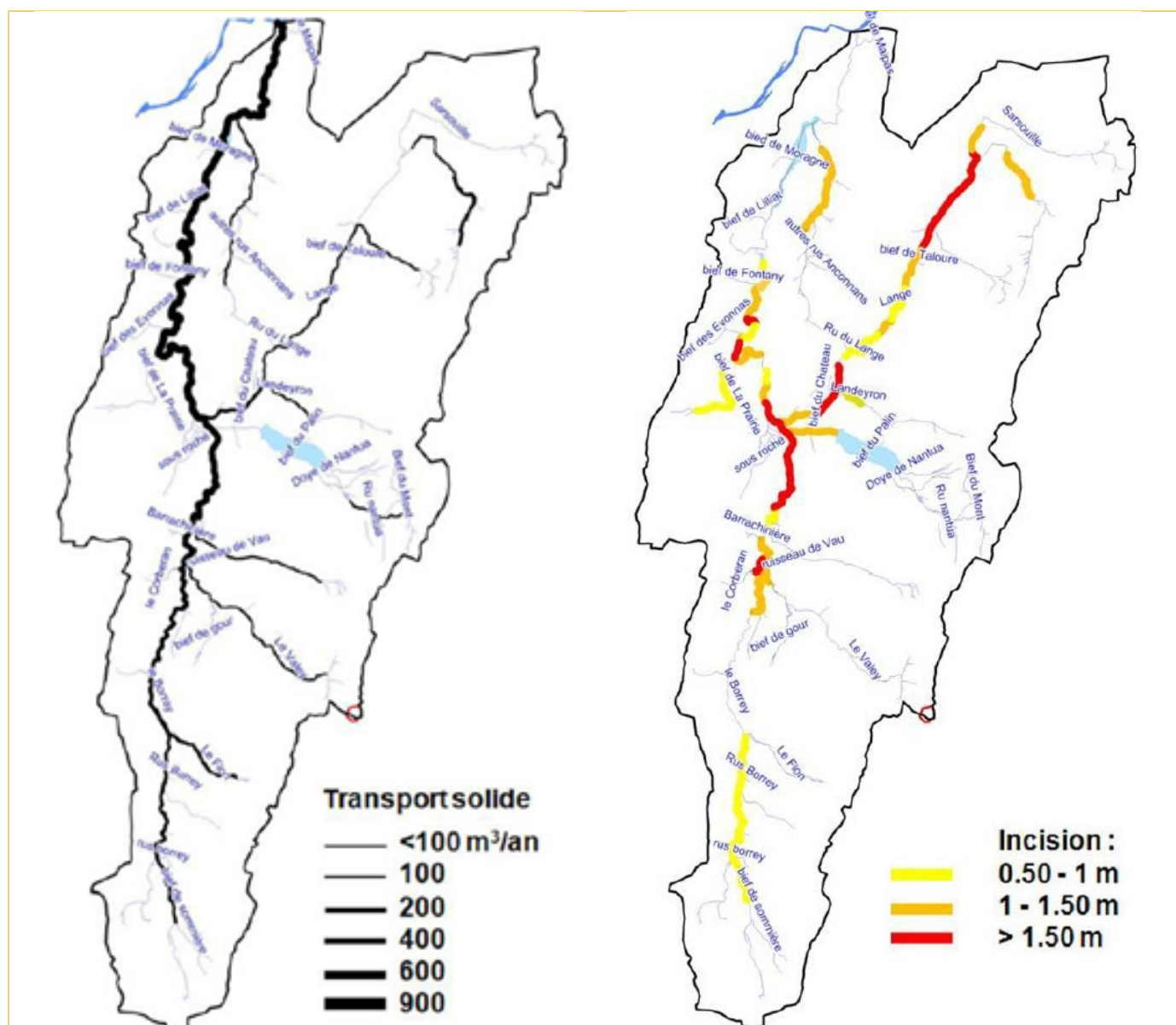
Représentation de la capacité de transport solide des cours d'eau du bassin versant
