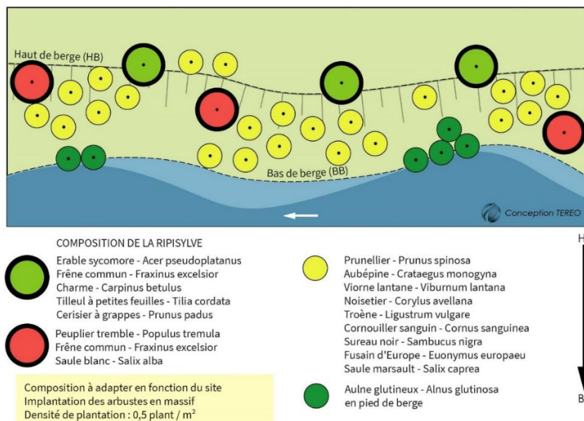
MODULE DE PLANTATION D'UNE ripisylve ligneuse
