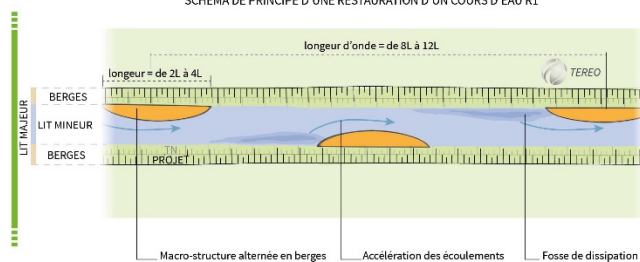
SCHEMA DE PRINCIPE D'UNE RESTAURATION D'UN COURS D'EAU R1
