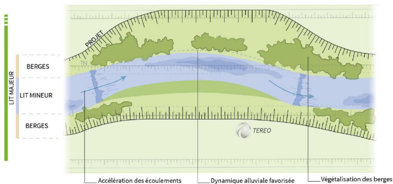
SCHEMA DE PRINCIPE D'UNE RESTAURATION D'UN COURS D'EAU R2
