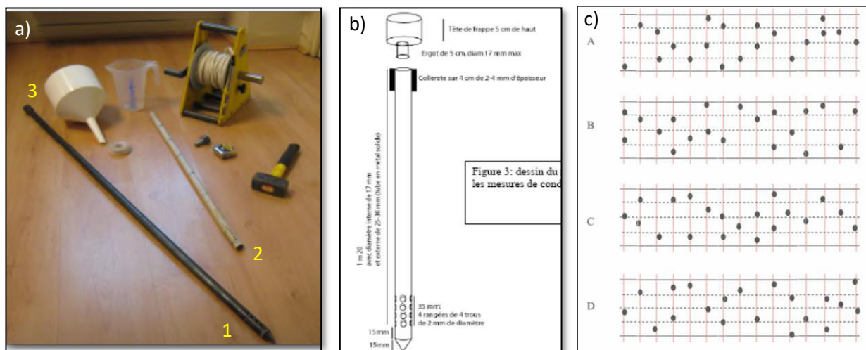
(a) Matériel nécessaire pour la mesure de la conductivité hydraulique (1 : pipe d'injection ; 2 : tube gradué pour mesurer le niveau ; 3 : entonnoir d'un litre pour injecter et mesurer le temps de transfert dans le lit), (b) schéma de la pipe d'injection et (c) exemple de positionnement des points de mesure sur quatre transects
