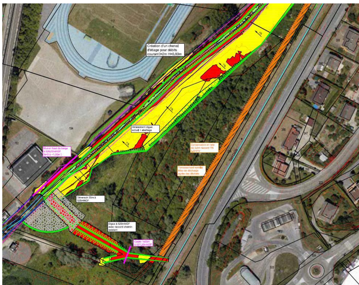
Vue en plan de la zone d'écêtement des crues proposée – ZEC 6
